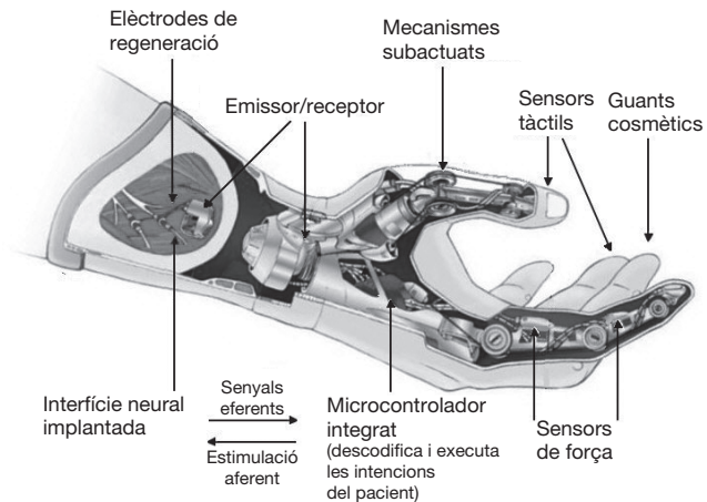
FIGURA 23. La mà bionica Cyberhand.
