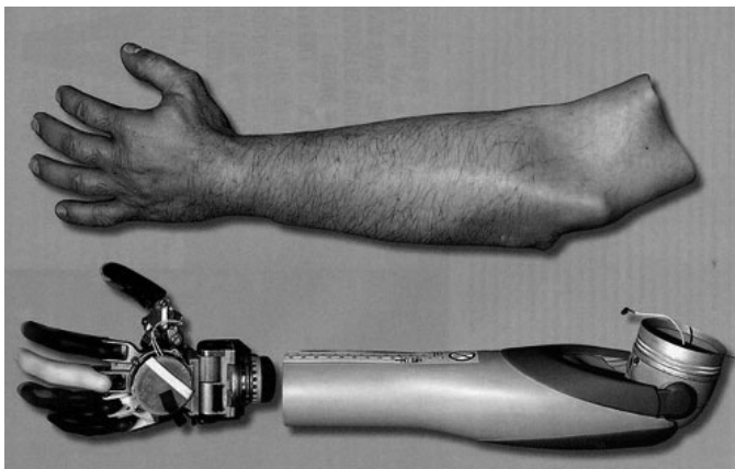
FIGURA 18. Braç ortopèdic robotitzat amb un recobriment mimètic de silicona.
