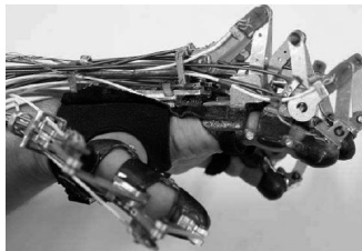
FIGURA 19. Ortesi destra experimental.
