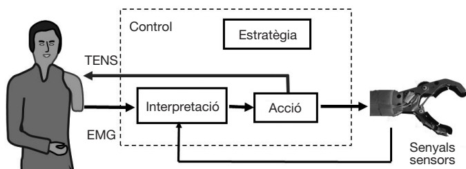
FIGURA 25. Pròtesi amb control EMG i retroalimentació de la força de pressió TENS.
