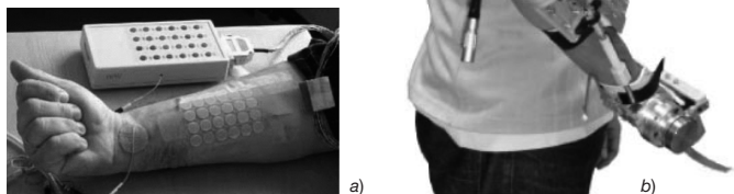
FIGURA 26. Compensació del tremolor patològic: a) amb EEF i b) amb exosquelet.
