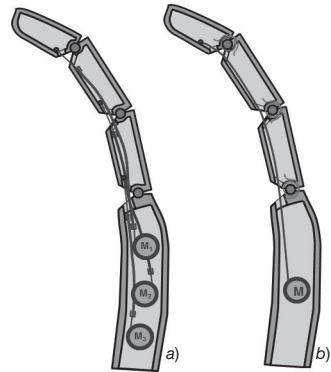
FIGURA 17. Dit amb tres articulacions amb: a) actuadors independents i b) estructura subactuada.
